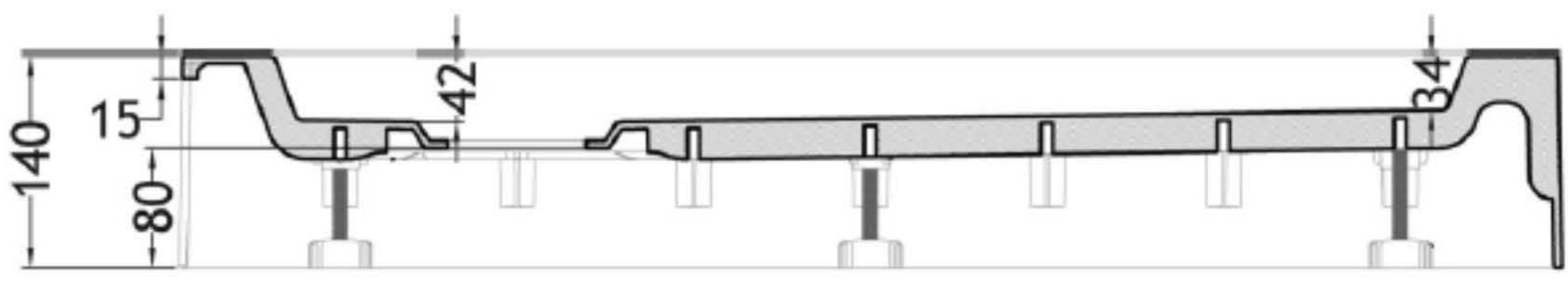
A-A
